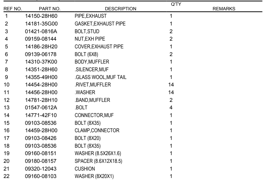
FIG.163A (1-B-15) MUFFLER
