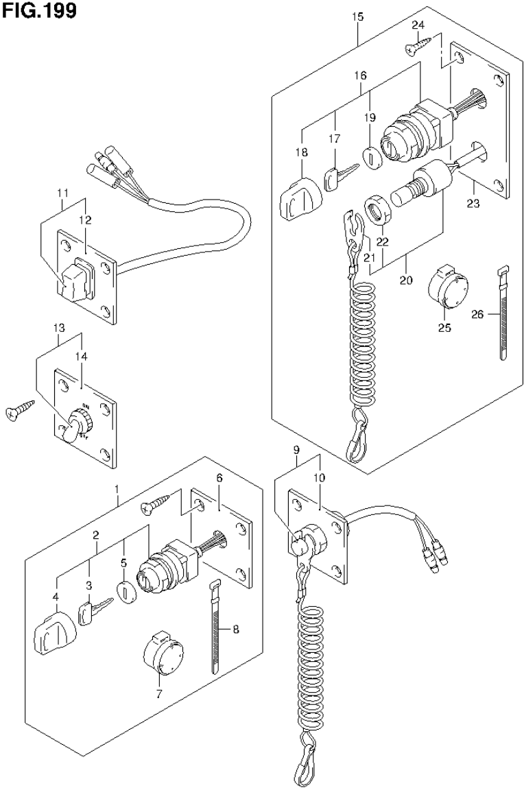
DF90A E01 013_199 OPT:SWITCH
