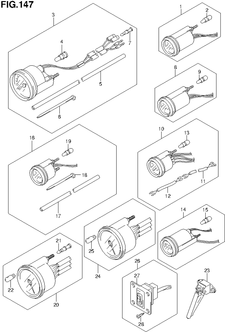
FIG.147 (2-C-13) OPT:METER (DF70A E1)
