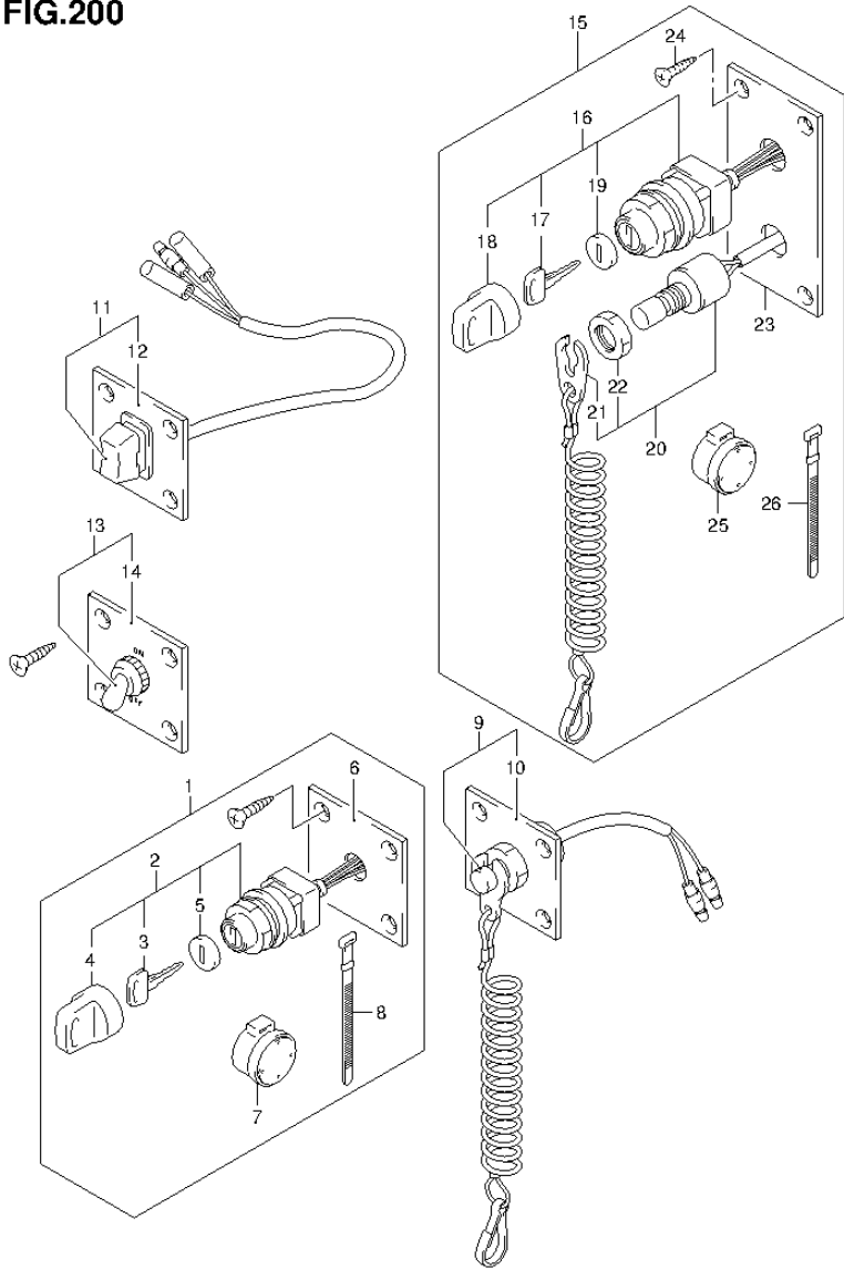
DF90A E01 013_200 OPT:SWITCH
