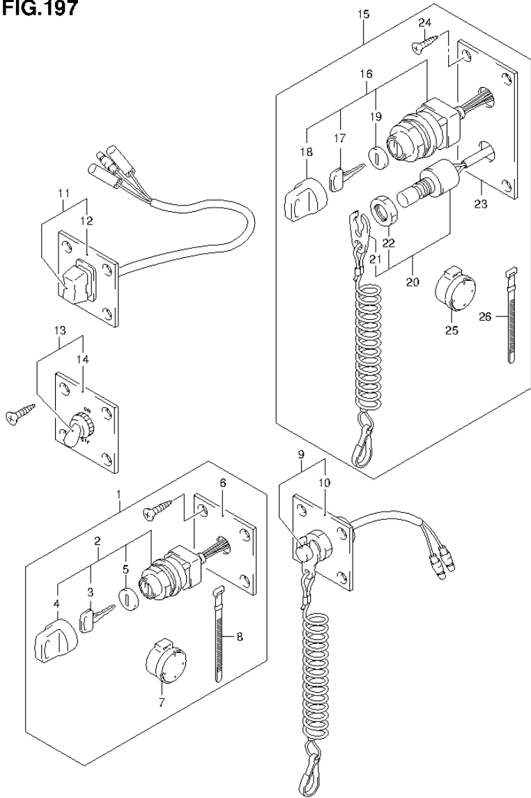
DF90A E01 013_197 OPT:SWITCH
