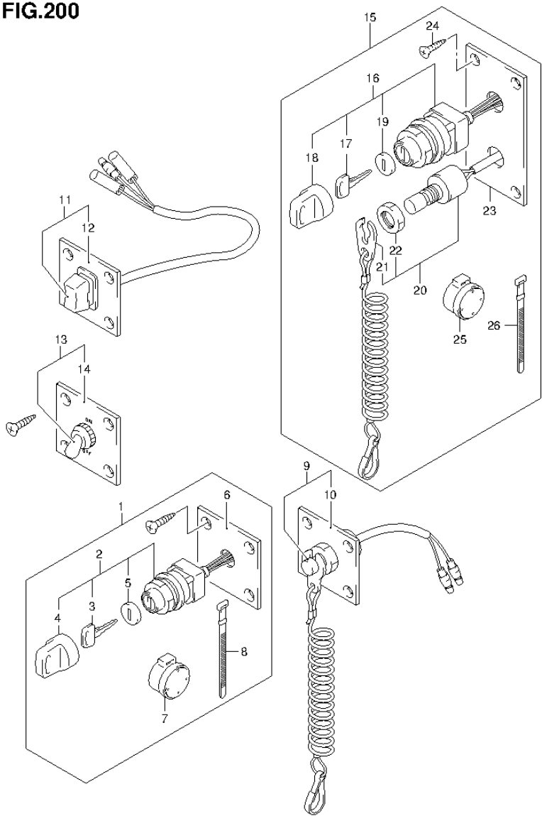
FIG.200 (2-I-14) OPT:SWITCH (DF90A E1)
