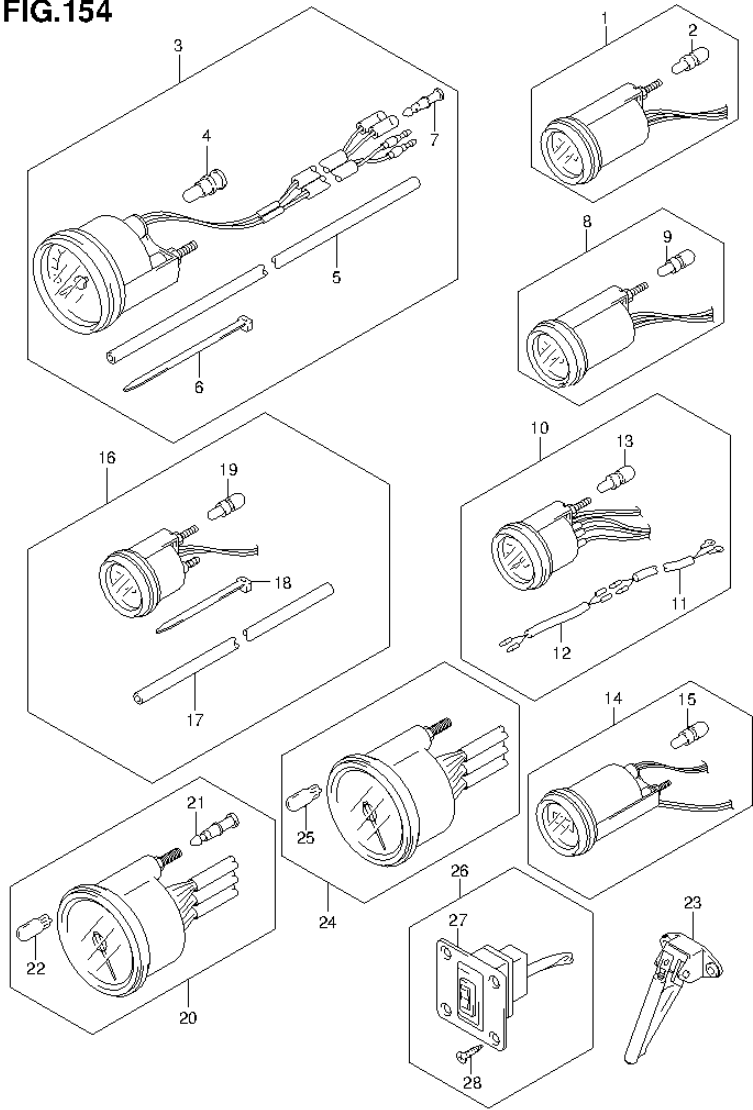
DF90A E01 013_154 OPT:METER
