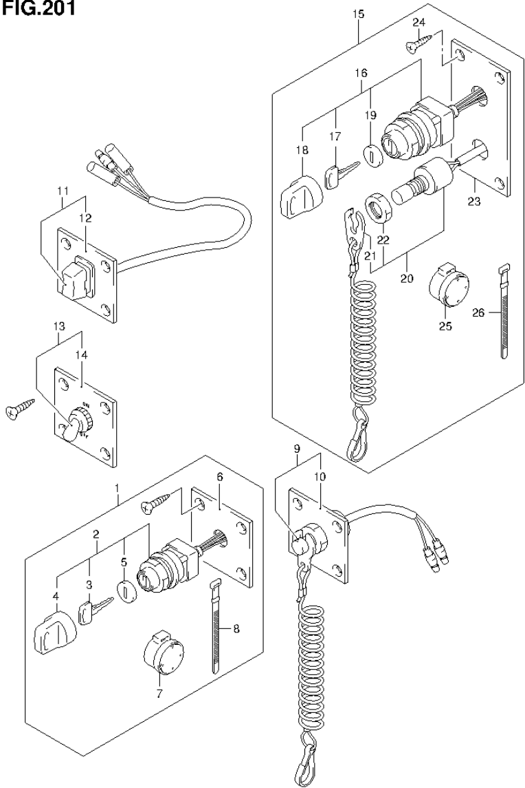
DF90A E01 013_201 OPT:SWITCH
