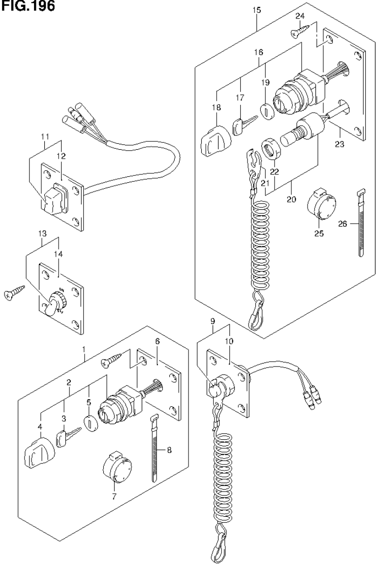
DF90A E01 013_196 OPT:SWITCH
