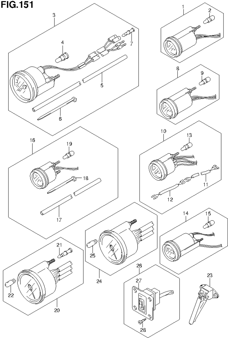
FIG.151 (2-D-7) OPT:METER (DF80A E1)
