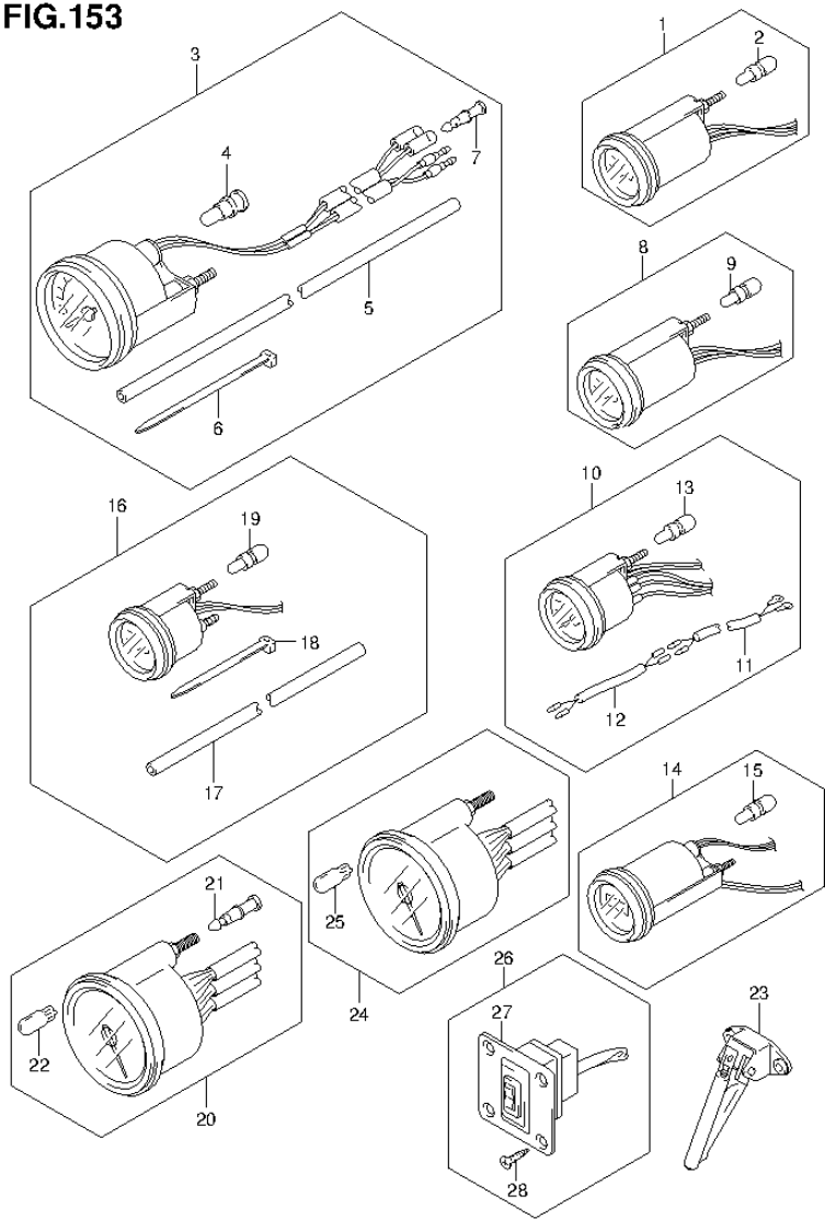
FIG.153 (2-D-11) OPT:METER (DF90A E1)
