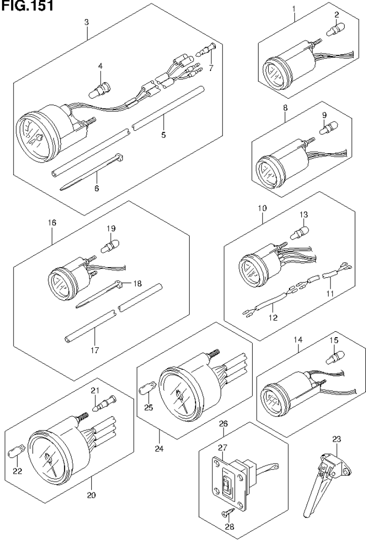
DF90A E01 013_151 OPT:METER
