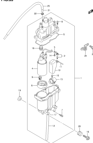
DF80A E01 013_005 FUEL VAPOR SEPARATOR
