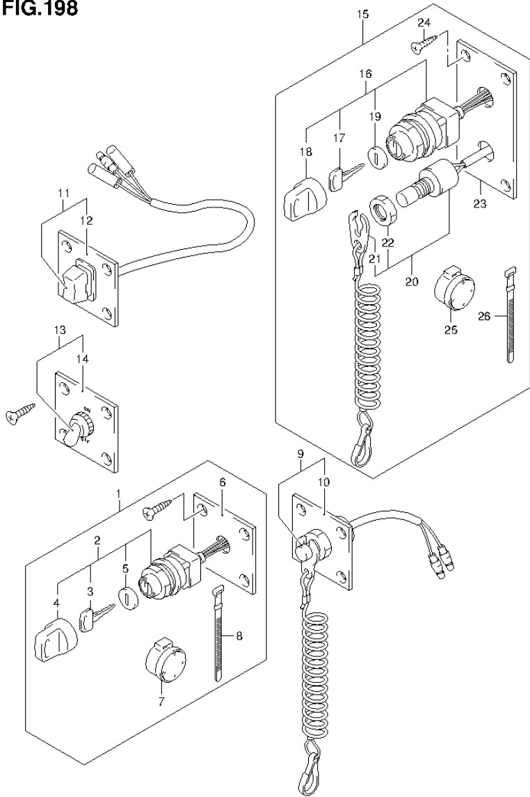
DF90A E01 013_198 OPT:SWITCH
