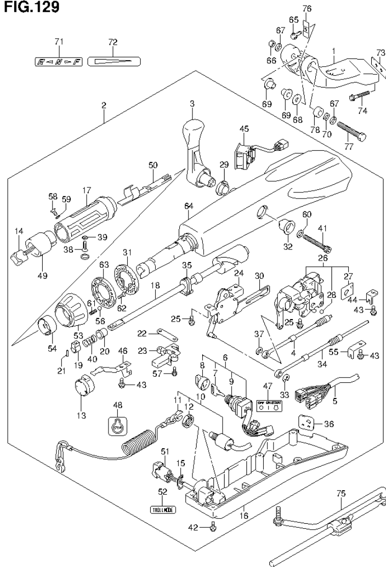
DF90A E01 013_129 TILLER HANDLE
