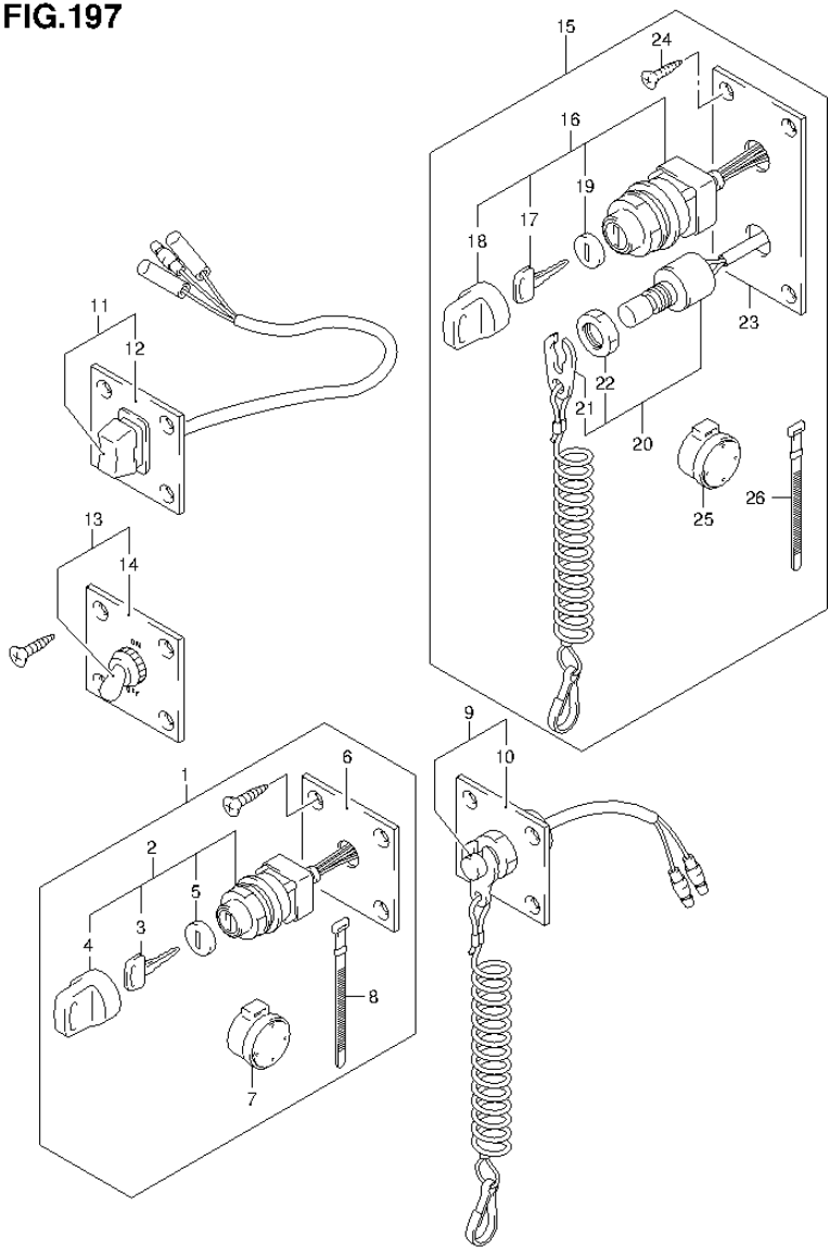
FIG.197 (2-I-8) OPT:SWITCH (DF70A E40)
