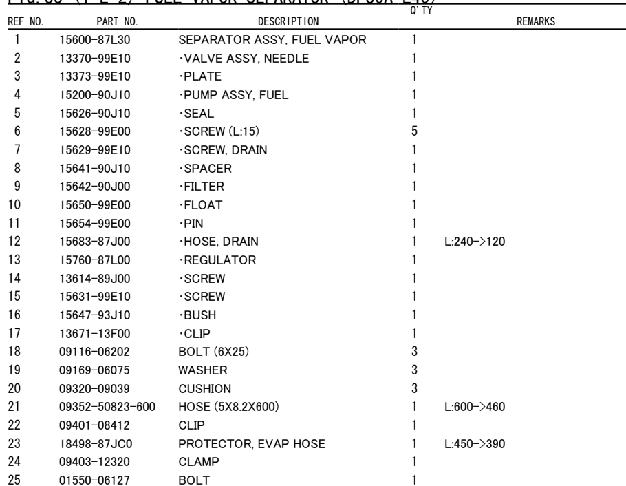
FIG. 33 (1-E-2) FUEL VAPOR SEPARATOR (DF80A E40)
