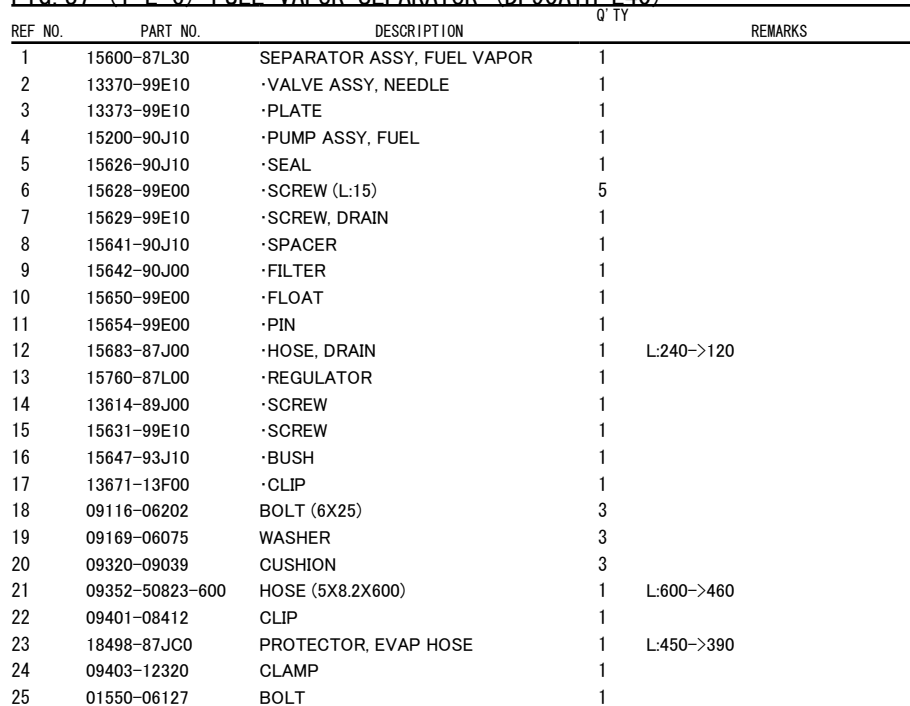
FIG. 37 (1-E-6) FUEL VAPOR SEPARATOR (DF90ATH E40)
